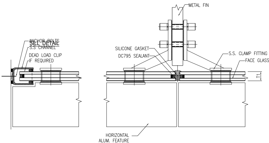
JAMB DETAIL
