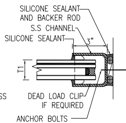
JAMB DETAIL
